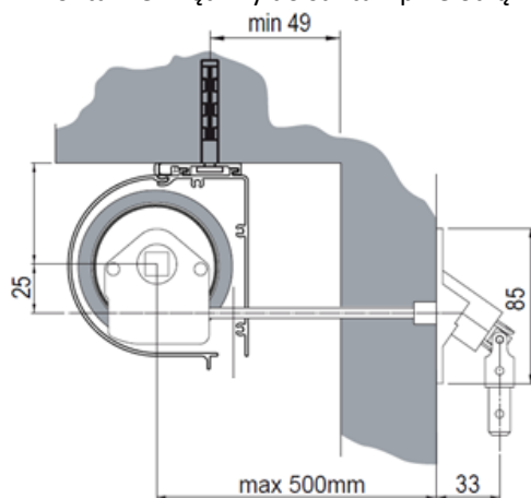
Montaż zewnętrzny do sufitu z przelotką
