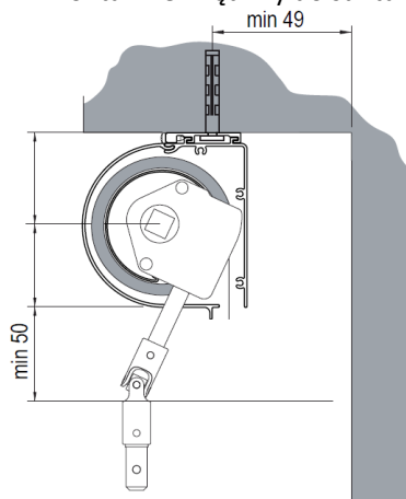
Montaż wewnętrzny do sufitu
